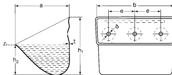
Stalen Columbus elevatorbekera (afmetingen in mm)
