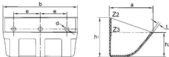
Kunststof elevatorbekers type D (afmetingen in mm)
