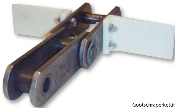
Gootschrapperketting met kunststof meenemers
