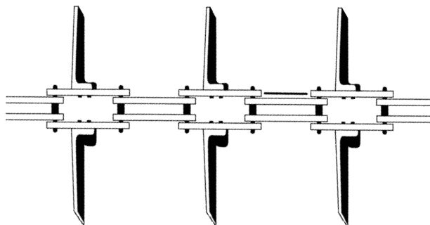
V.A.V. gootschraperketting (afmetingen in mm)
