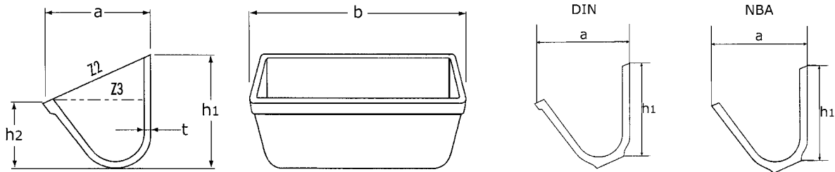
Monocast GSM elevatorbekers NBA-serie (afmetingen in mm)
