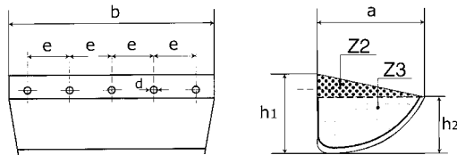
Starco elevatorbekers in gelaste uitvoering (afmetingen in mm)
