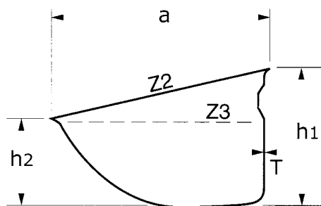
Starco elevatorbekers uit kunststof (afmetingen in mm)
