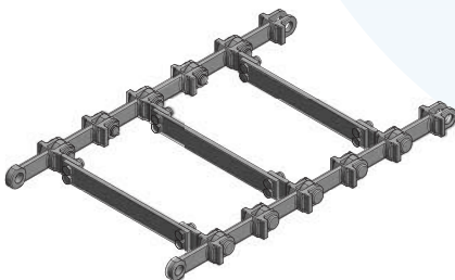
Dubbelstreng met traverse
