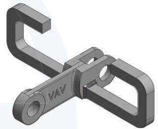
"O"-vorm voor verticaal transport
