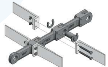
Met eenvoudig te monteren kunststof meenemers
